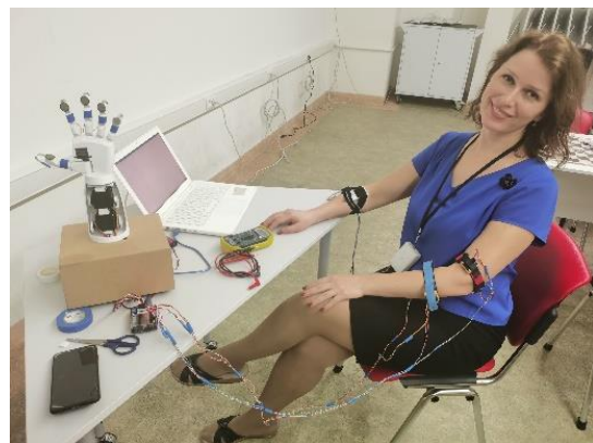
Рисунок 14. Тестирование системы обратной связи
